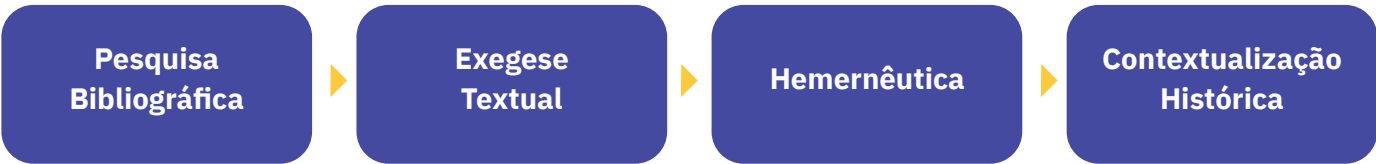
Figura 2: Fluxograma Metodológico
